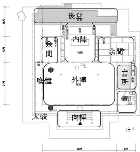
図6 興真寺平面図(高松花作成 一部改変)
